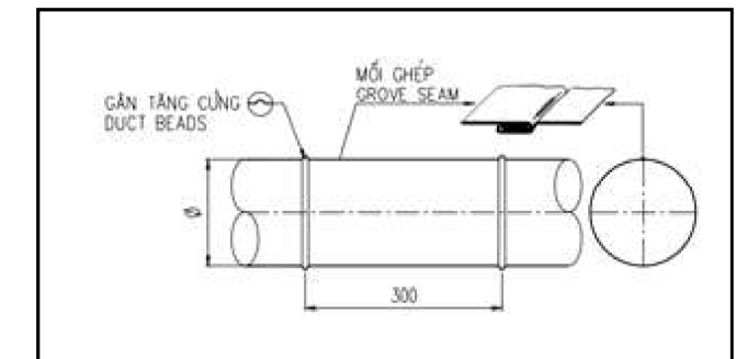
ỐNG GIÓ TRÒN TRƠN (truyền thống)
